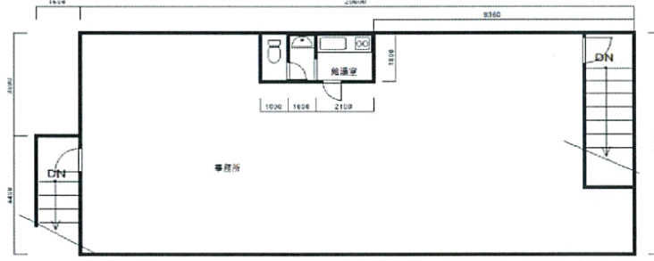
2階 平面図
